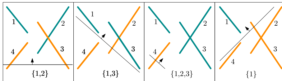
Abbildung 23: Shattering einer Menge von 4 Segmenten mit nur einer Überschneidung. Es ist abgebildet, wie die Teilmengen \{1, 2\} , \{1, 3\} , \{1, 2, 3\} , und \{1\} Abgedeckt werden können. Alle weiteren Teilmengen folgen analog.
