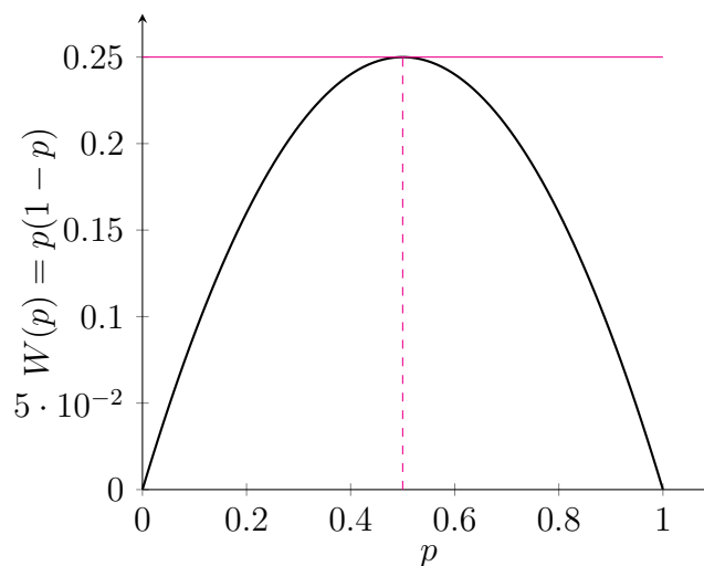
Abbildung 12: Die Wahrscheinlichkeitsfunktion W(p) = p(1 - p) .
