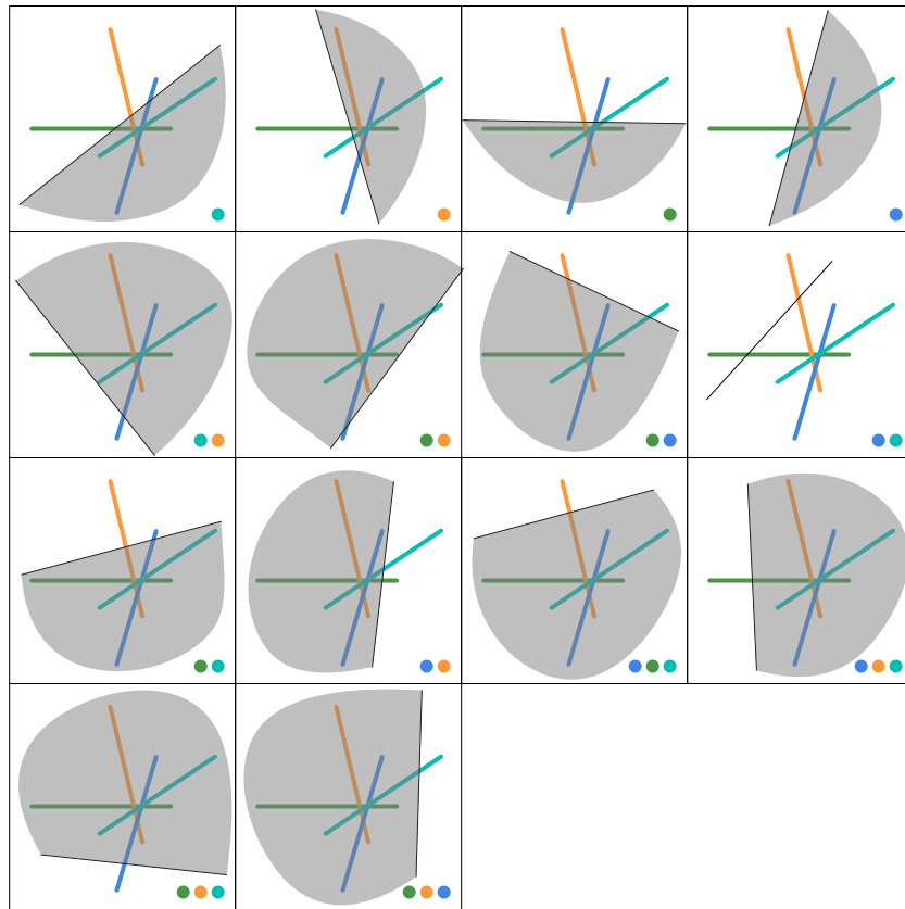
Abbildung 22: Eine Anordnung von vier Streichhölzern, sodass jede Teilmenge der Streichhölzer von dem großen Papier (grau) bedeckt wird.
